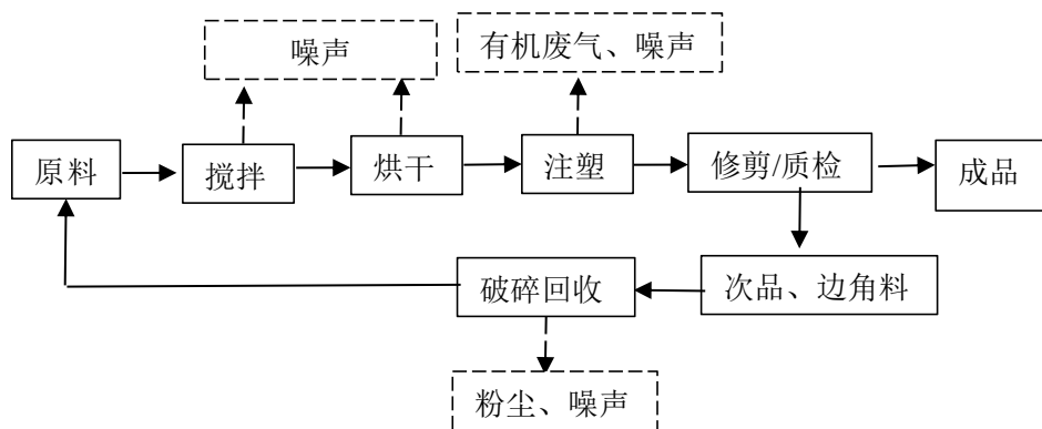
图 2-2 原项目生产工艺流程图
