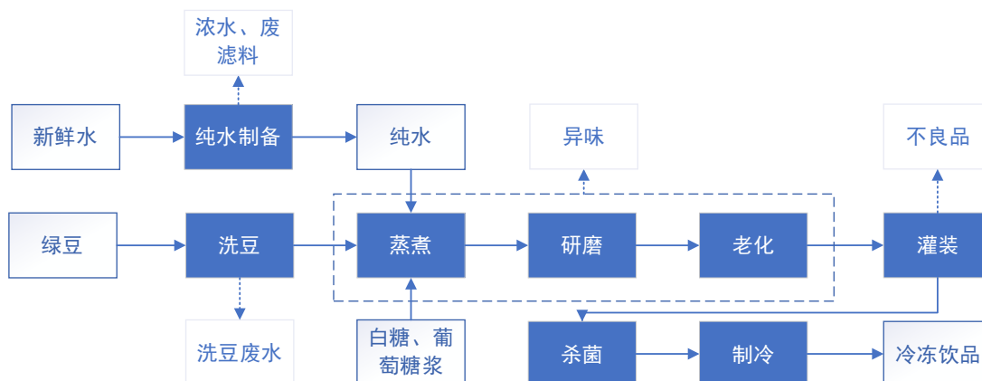
图3 冷冻饮品工艺流程图
