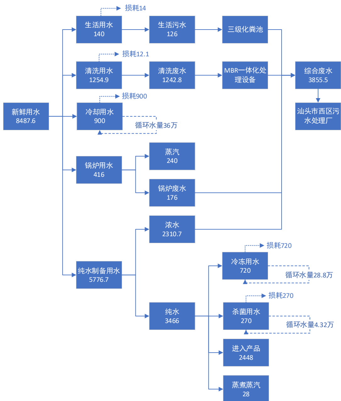
图1 水平衡图（单位：t/a）
